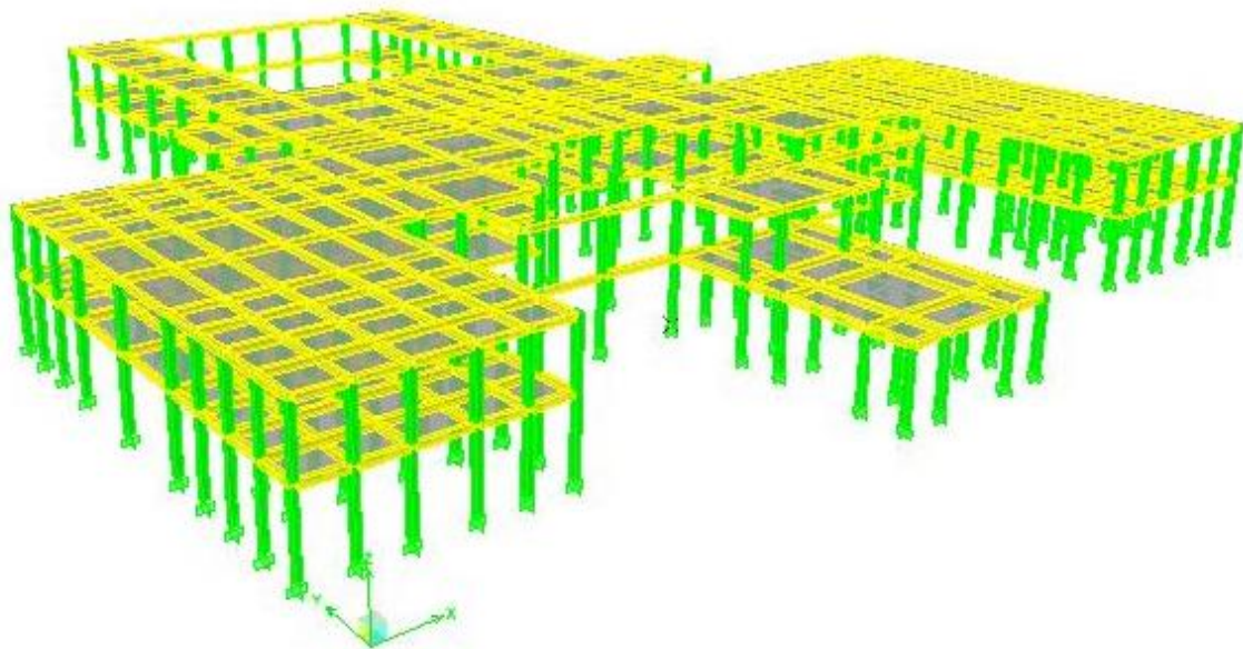
Gambar 4.1: Model Bangunan
